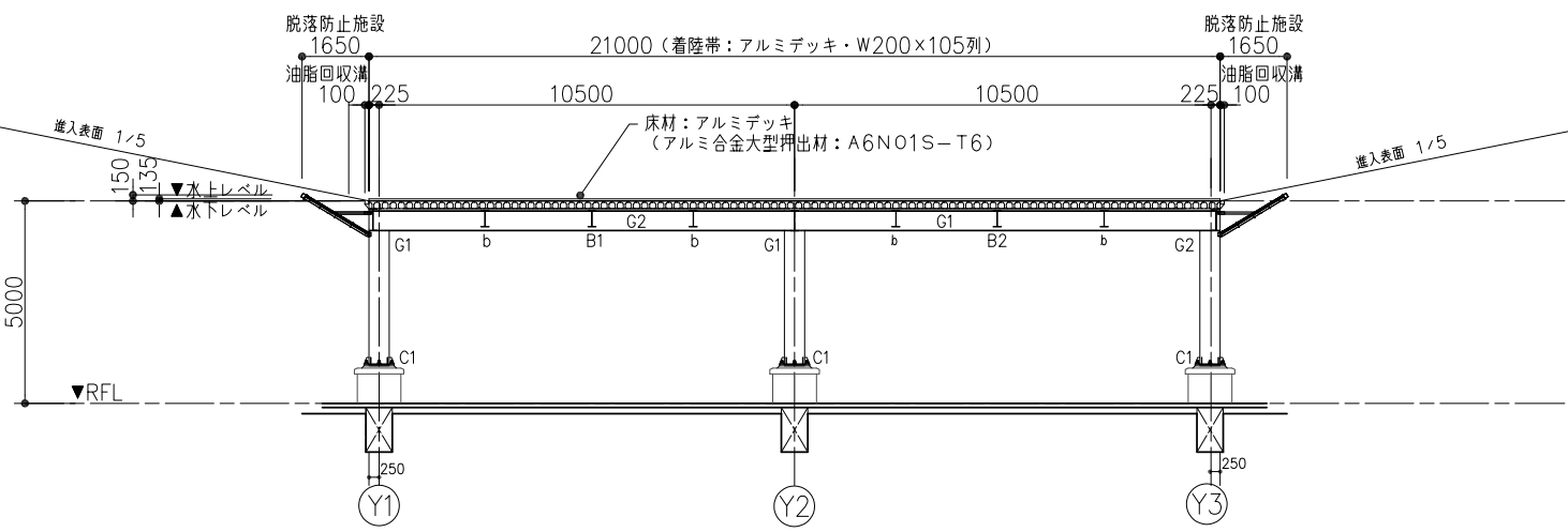
Y-Y断面図 1:200
