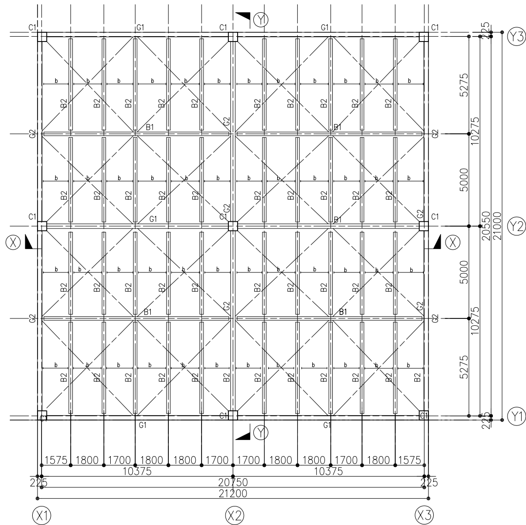
梁伏図 1:200
