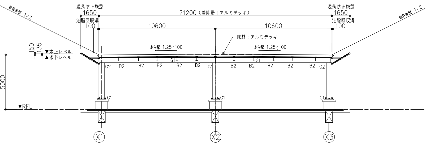
X-X断面図 1:200
